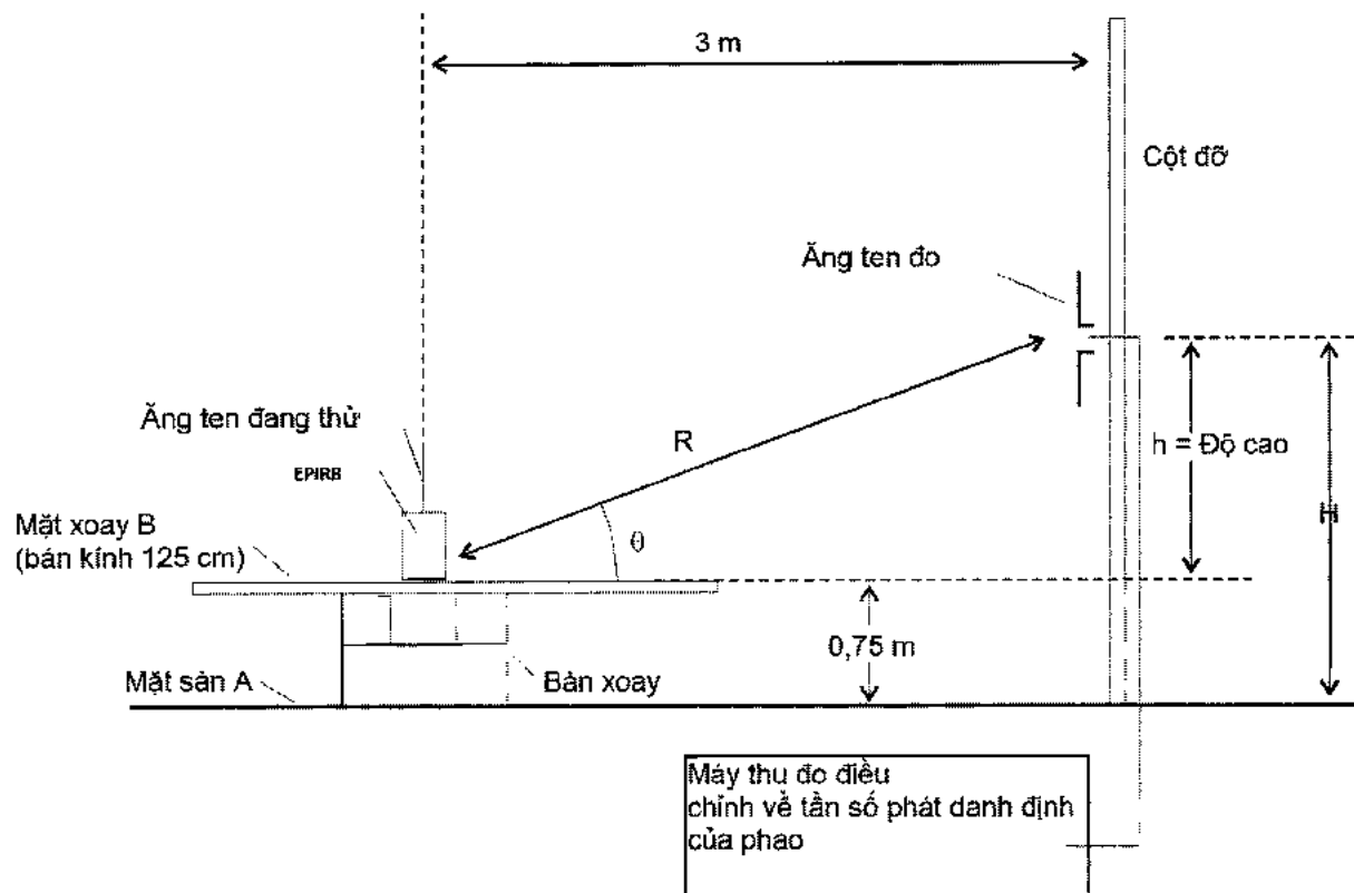
Hình 2 - Thiết lập đo kiểm
