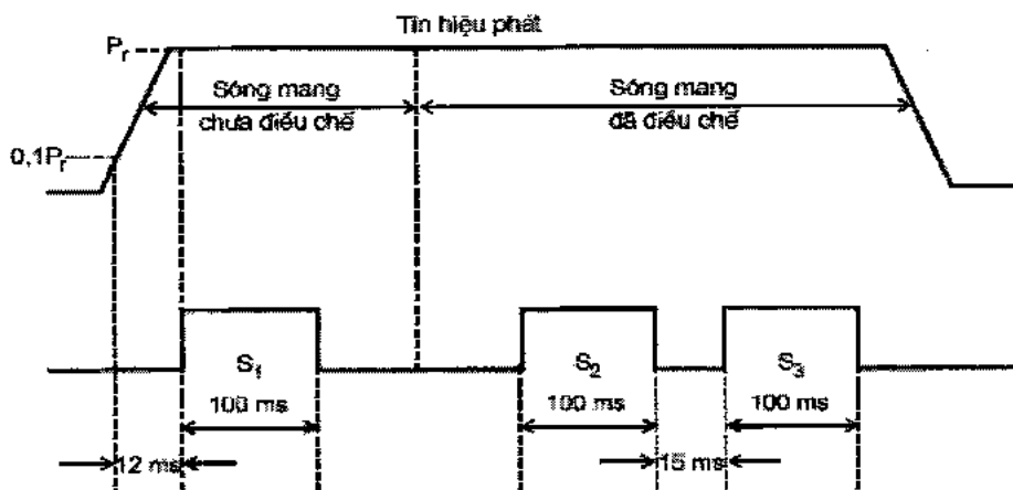
Hình 5 - Thời gian đo tần số đặc trưng
